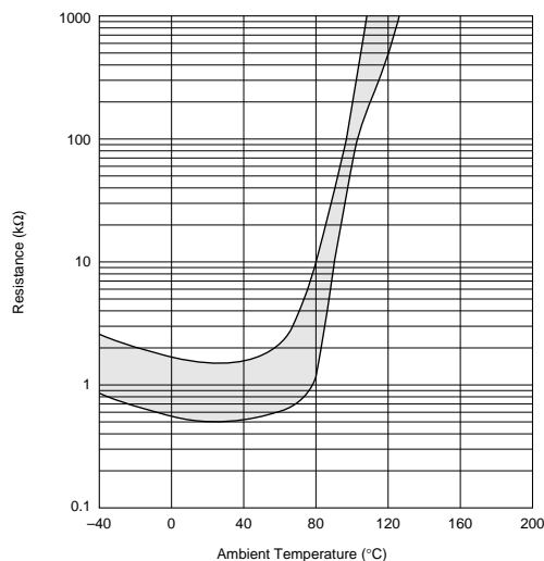
PRF15BE102RB6RC
