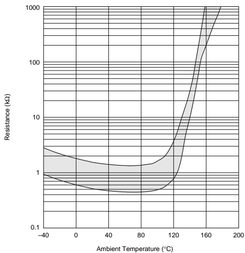
PRF15AR102RB6RC
