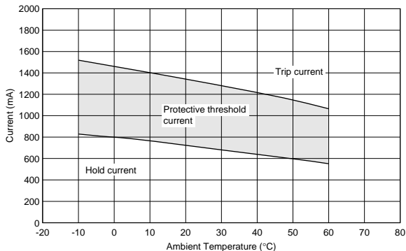
PTGL07ARR47M1B51B0
