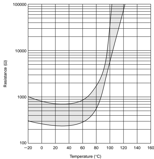
PRF18BD471RB5RB
