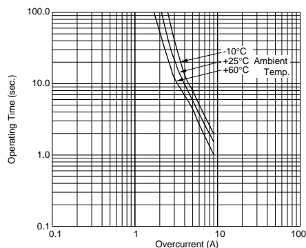
PTGL12AR0R2M1B51B0
