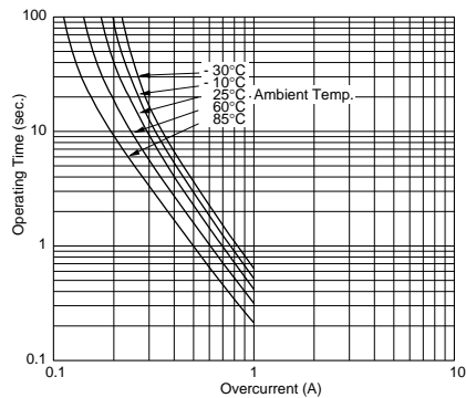
PTGL05AS270K6B51B0
