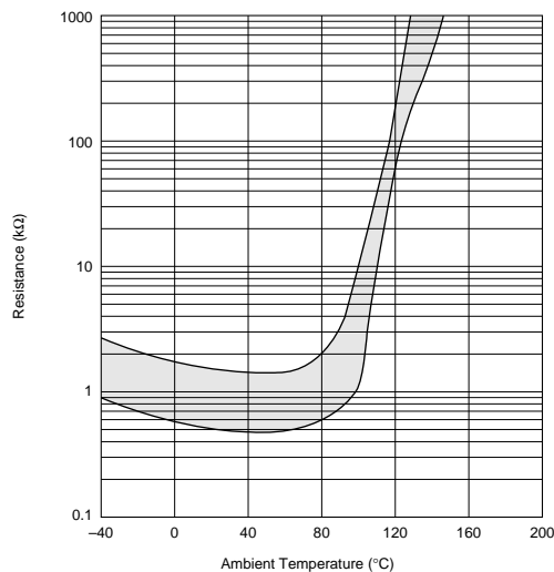
PRF15BC102RB6RC
