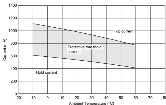
PTGL06AR0R8M1B51B0
