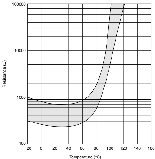
PRF18/21BD471Q Type
