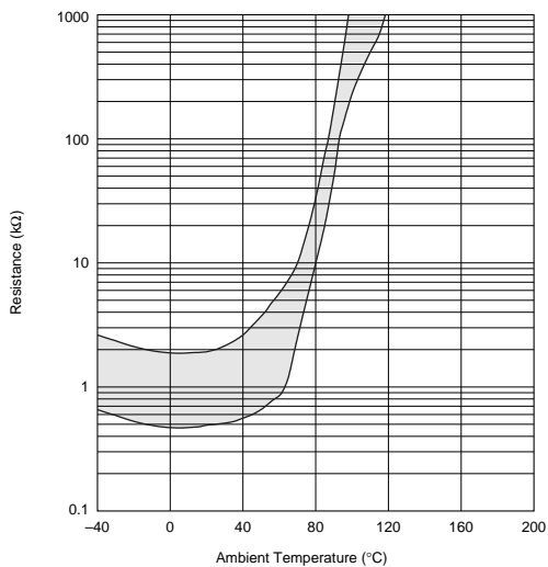
PRF15BF102RB6RC
