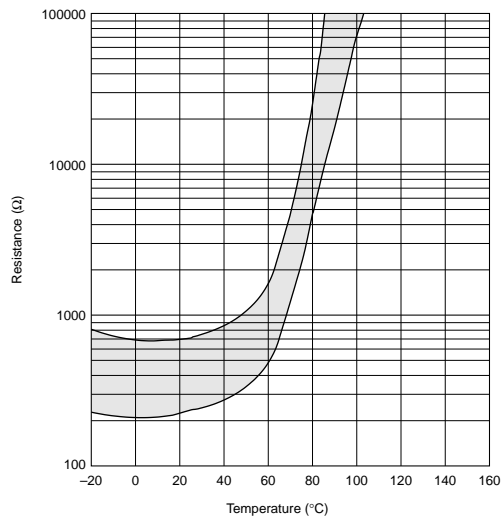
PRF18BF471Q Type
