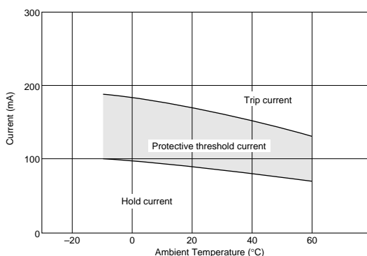
PTGL07AR650H8B52B0
