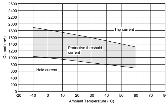
PTGL09ARR33M1B51B0
