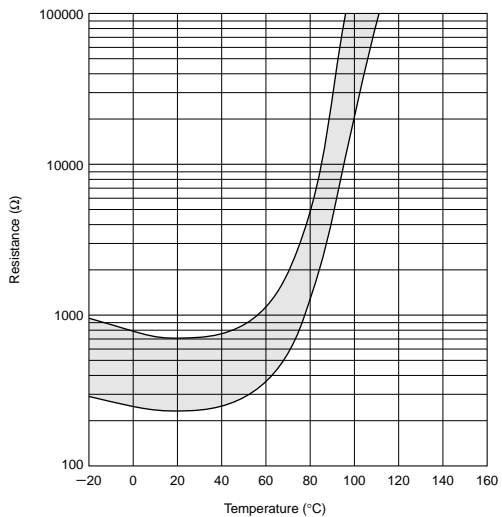
PRF18/21BE471Q Type
