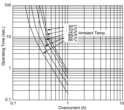
PTGL04AS100K3B51B0
