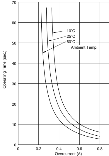
PTGL09AR220M6B52B0
