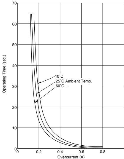
PTGL07AR700H8B52B0
