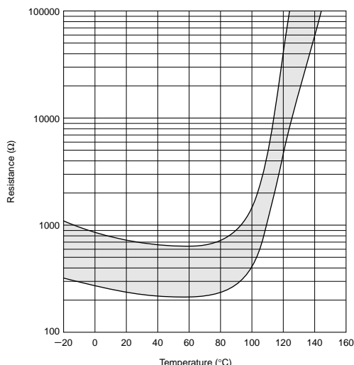
PRF18/21BB471Q Type
