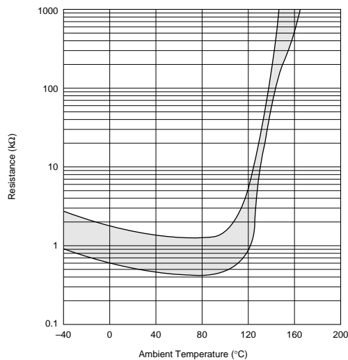
PRF15BA102RB6RC
