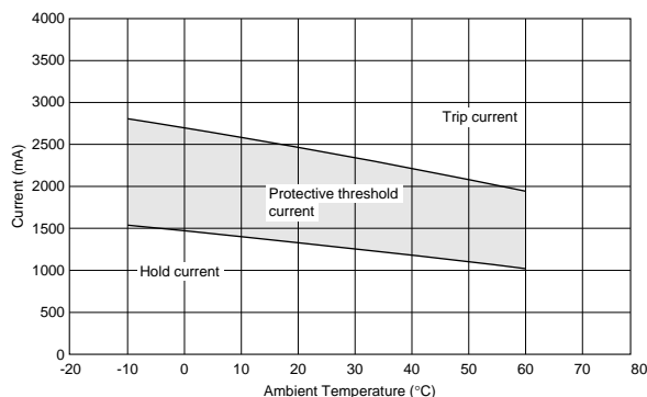
PTGL12AR0R2M1B51B0
