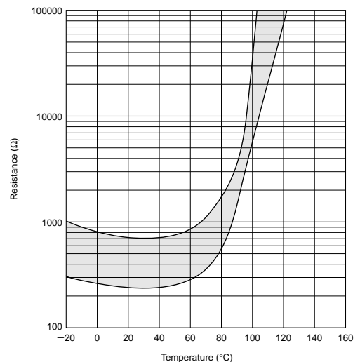
PRF18BD471RB5RB
