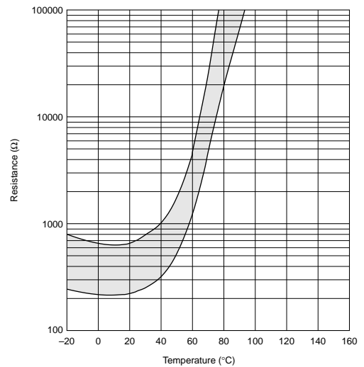
PRF18BG471Q Type
