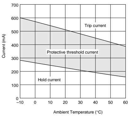
PRG18/21BC2R2M Type
