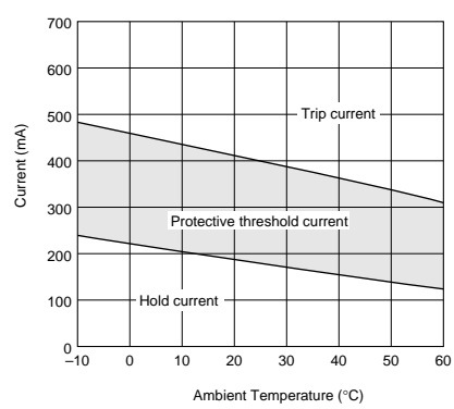
PRG18/21BC3R3M Type
