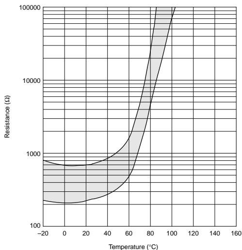
PRF18BF471Q Type
