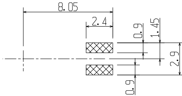
Recommendable P.C. Board layout 推奨基板レイアウト
